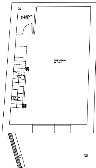
PLANTA SEMISOTANO.
