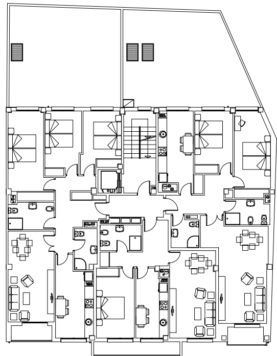
PLANTA PRIMERA.
