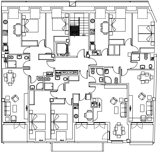
PLANTA BAJOCUBIERTA.
