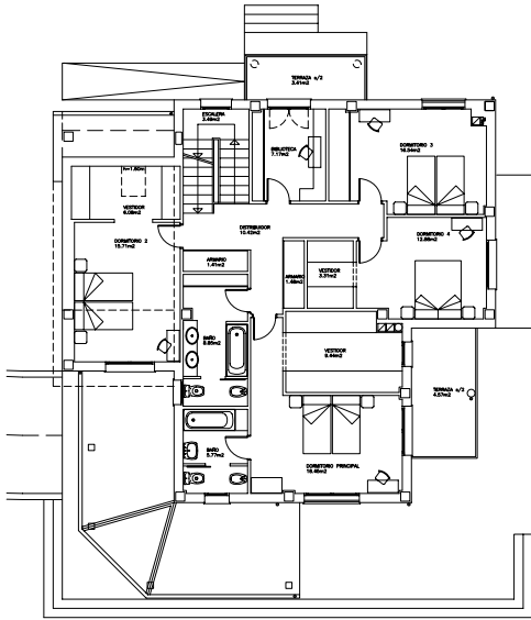
PLANTA PRIMERA.
