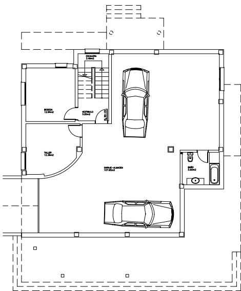
PLANTA SOTANO.
