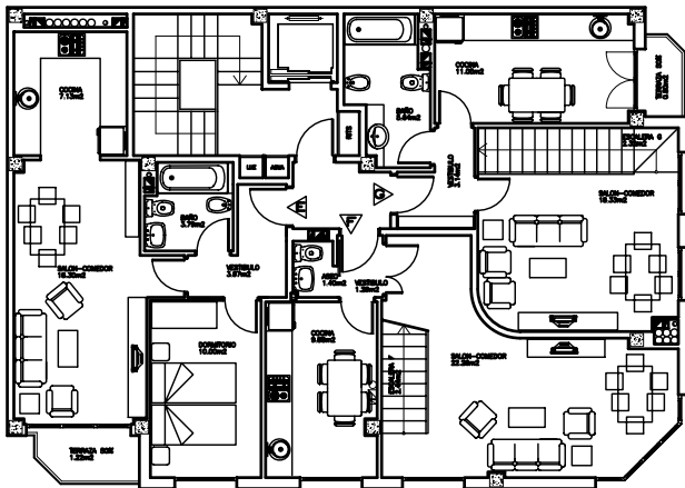
PLANTA SEXTA. DISTRIBUCION Y MOBILIARIO
