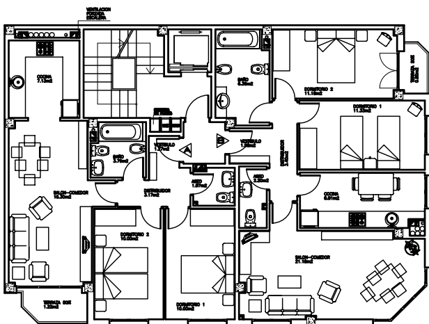
PLANTA TIPO. DISTRIBUCION Y MOBILIARIO
