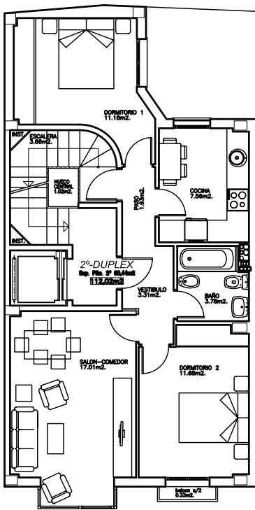
PLANTA SEGUNDA.DISTRIBUCION Y MOBILIARIO.
