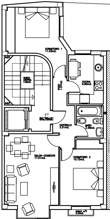
PLANTA PRIMERA. DISTRIBUCION Y MOBILIARIO.
