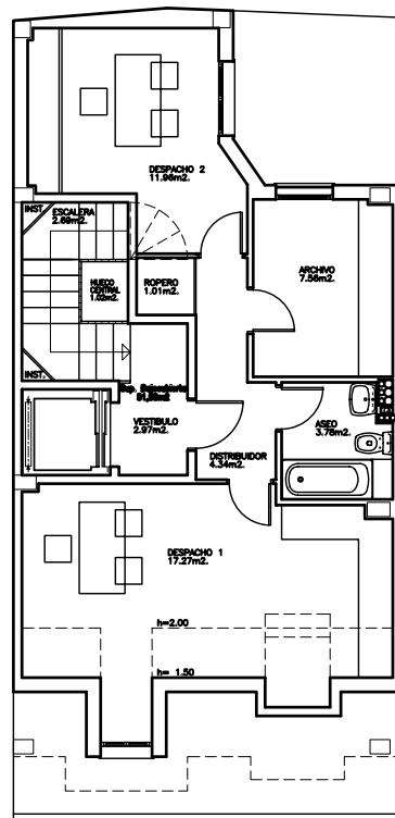
BAJOCUBIERTA. DISTRIBUCION Y MOBILIARIO.
