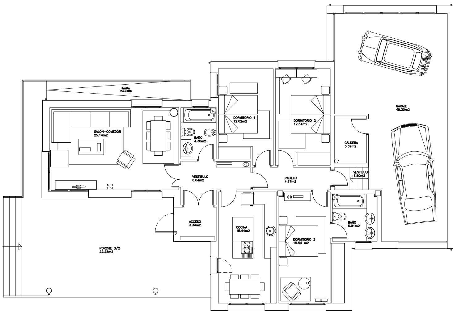
PLANTA BAJA.
