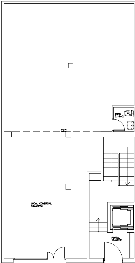
PLANTA BAJA.
