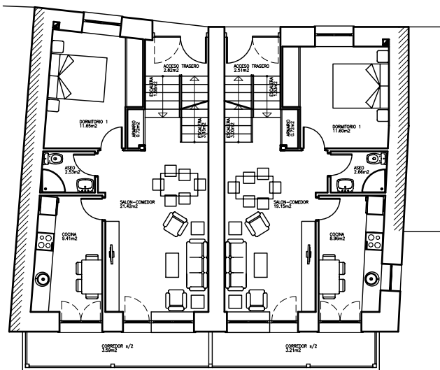
PLANTA PRIMERA.
