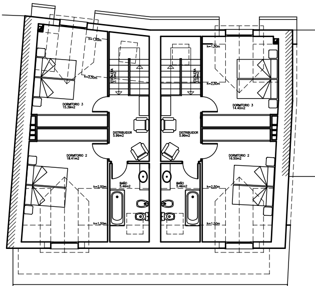
PLANTA BAJOCUBIERTA.
