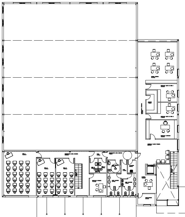
PLANTA PRIMERA, ALMACEN Y SERVIDOR
