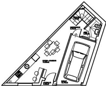
PLANTA BAJA.DISTRIBUCION Y MOBILIARIO
