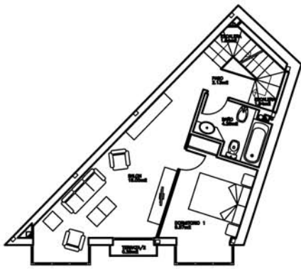
PLANTA PRIMERA.DISTRIBUCION Y MOBILIARIO
