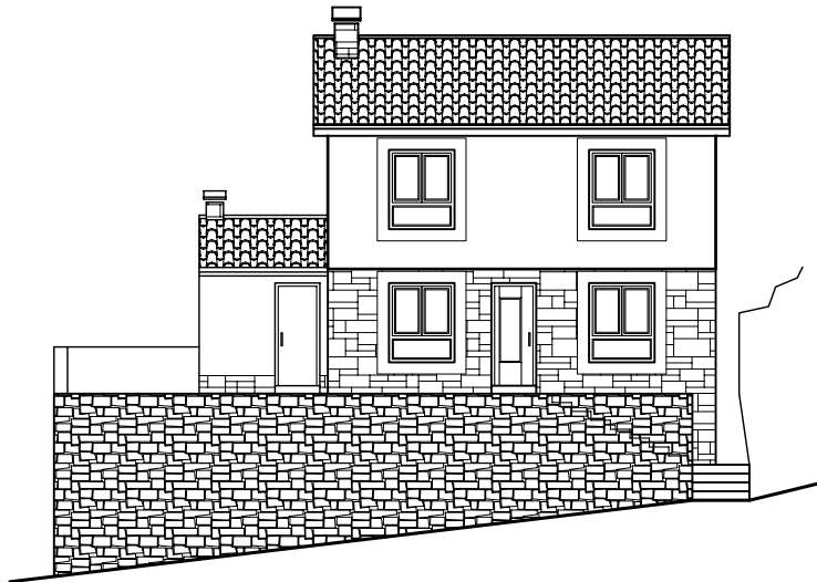
ALZADO PRINCIPAL.
