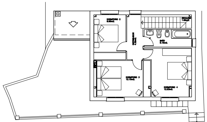
PLANTA PRIMERA.
