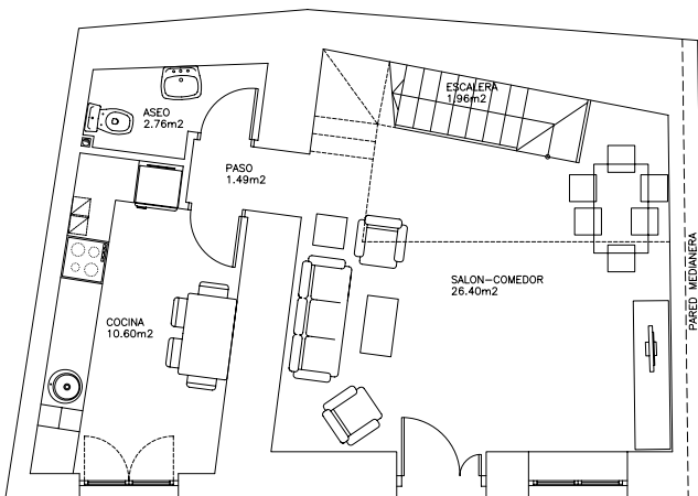
PLANTA BAJA.
