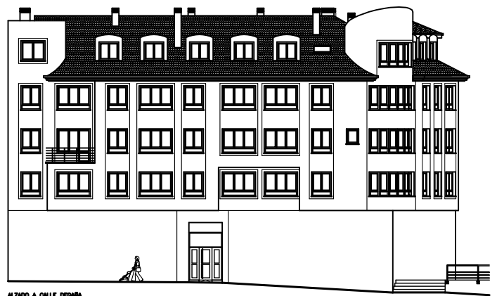
ALZADO A CALLE DEGAÑA
