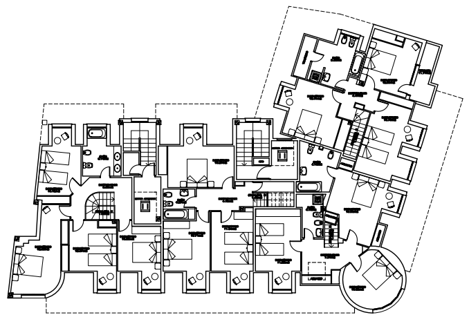
PLANTA BAJOCUBIERTA
