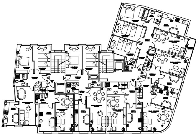
PLANTA TERCERA
