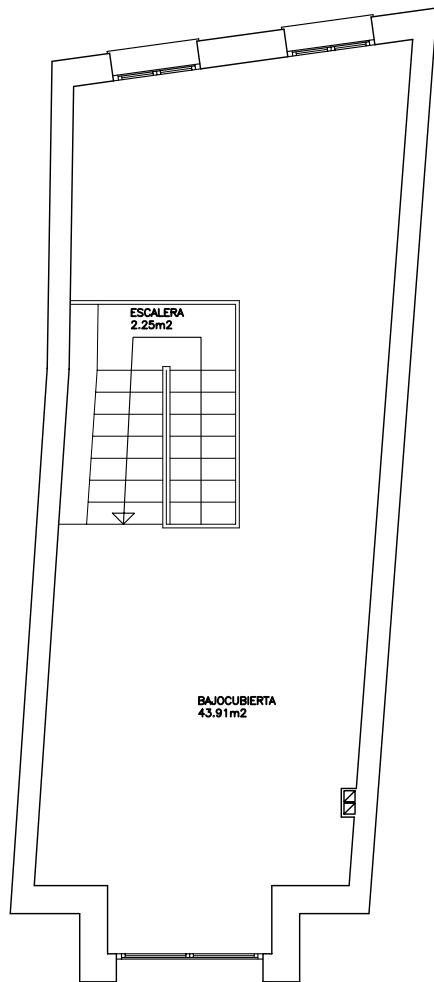
BAJOCUBIERTA.
