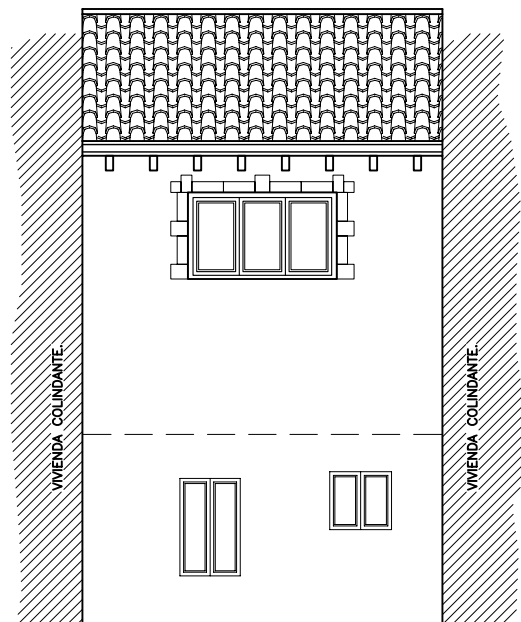
ALZADO POSTERIOR.
