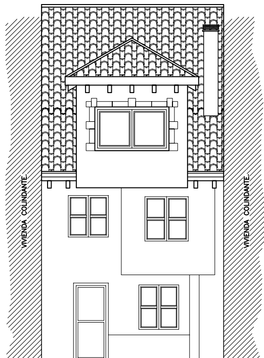
ALZADO PRINCIPAL.
