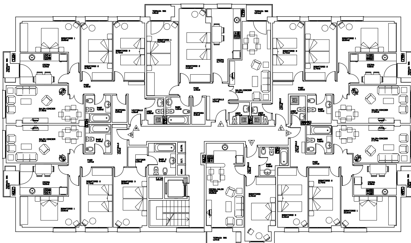
PLANTA TIPO.
