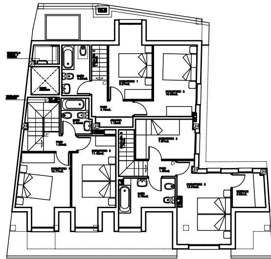
BAJOCUBIERTA. DISTRIBUCION Y MOBILIARIO
