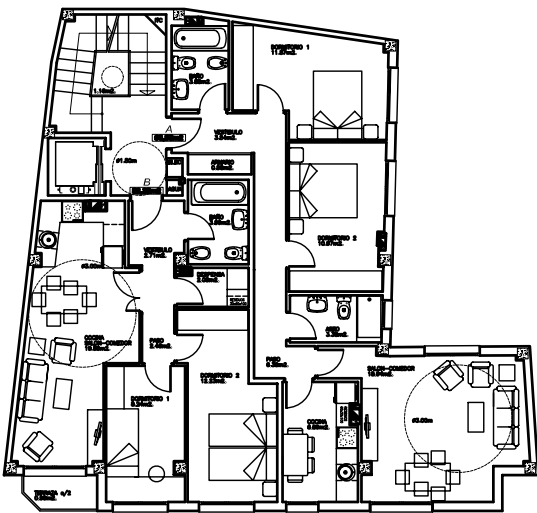
PLANTA PRIMERA Y SEGUNDA. DISTRIBUCION Y MOBILIARIO
