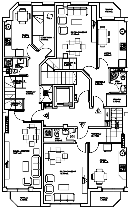
PLANTA QUINTA. DISTRIBUCION Y MOBILIARIO
