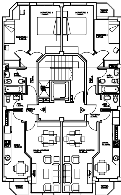
PLANTAS 2ª, 3ª Y 4ª. DISTRIBUCION Y MOBILIARIO
