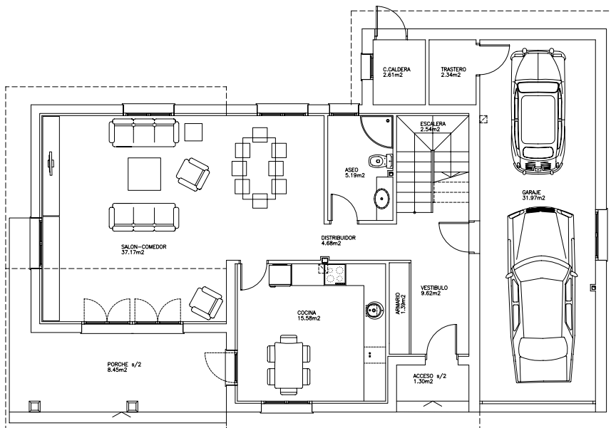
PLANTA BAJA.
