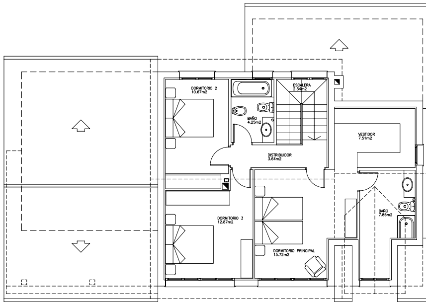
PLANTA PRIMERA.
