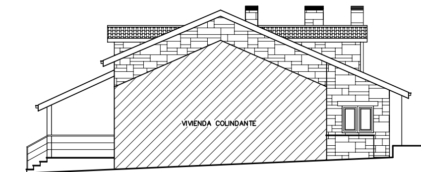
ALZADO LATERAL IZQUIERDO.
