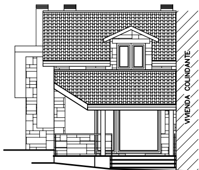
ALZADO POSTERIOR.
