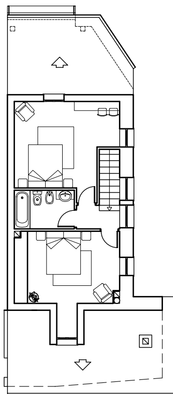
PLANTA BAJOCUBIERTA. DISTRIBUCIÓN Y MOBILIARIO.
