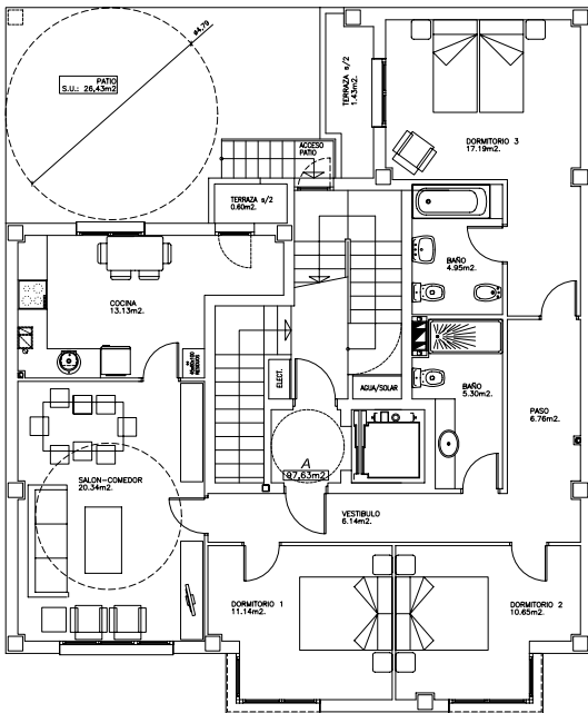
PLANTA PRIMERA.
