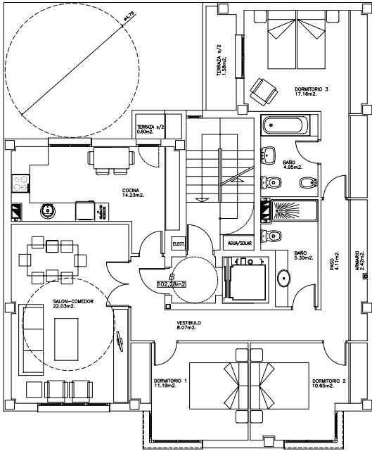
PLANTA SEGUNDA.
