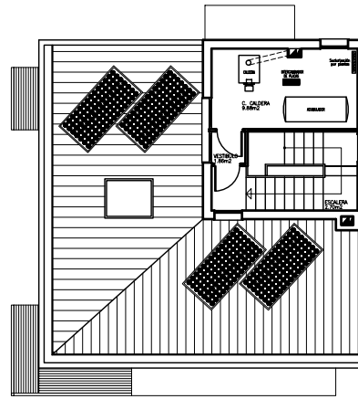
PLANTA CUBIERTA.
