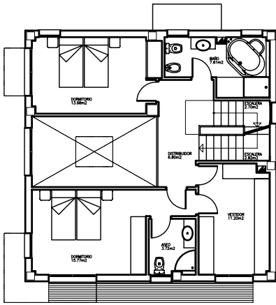
PLANTA PRIMERA.
