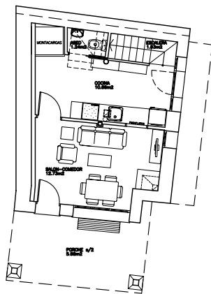
PLANTA SEMISOTANO.
