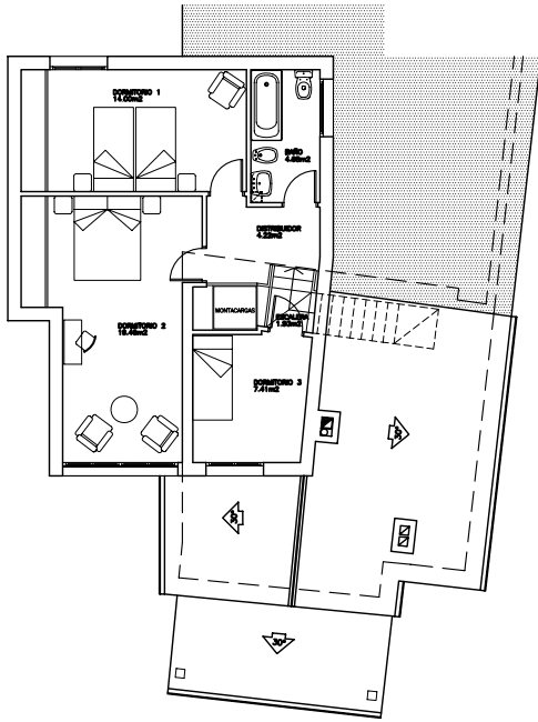
PLANTA PRIMERA.
